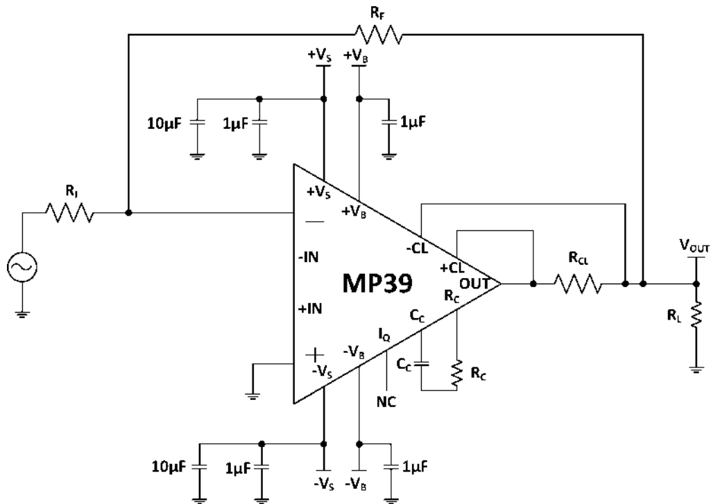
Figure 2: 代表的な回路図
