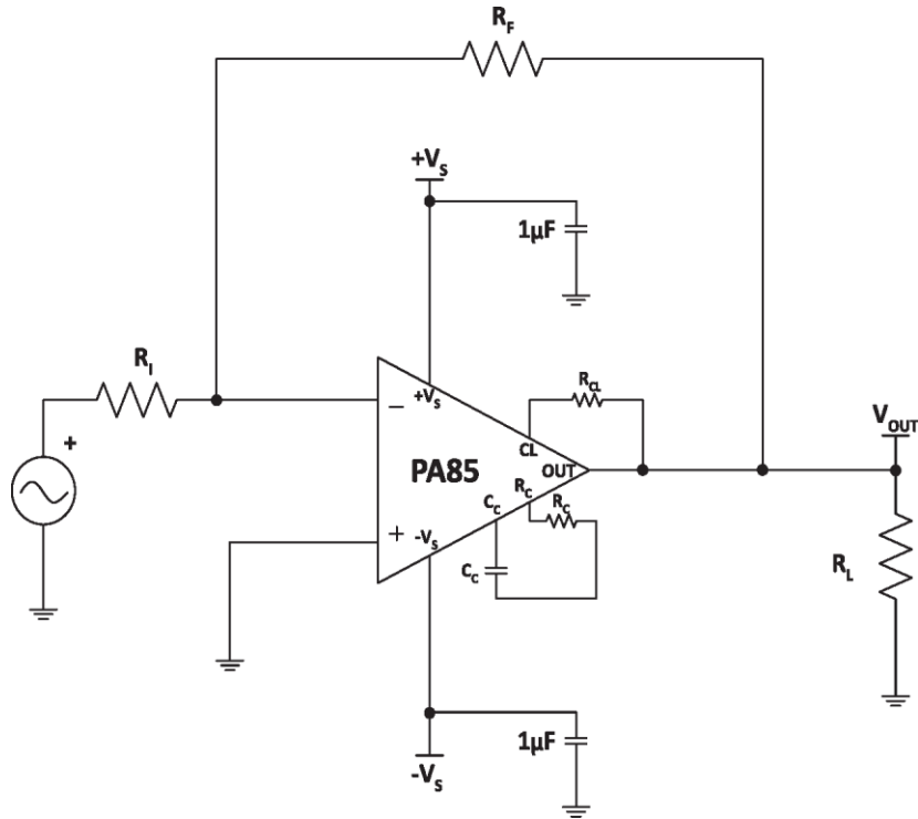
Figure 2: 代表的な接続図
