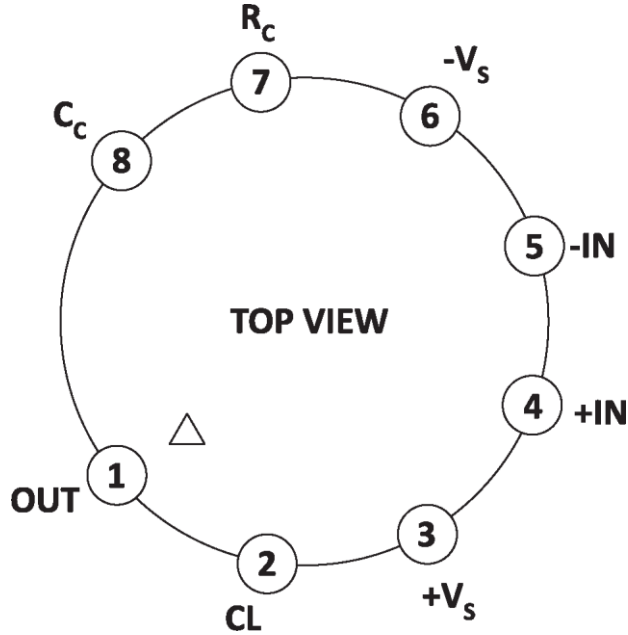
Figure 3: 外部接続
