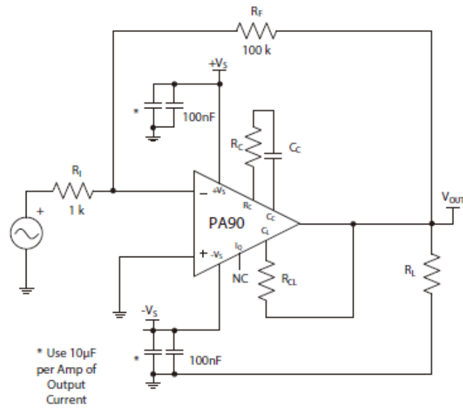
Figure 2: 代表的な接続図
