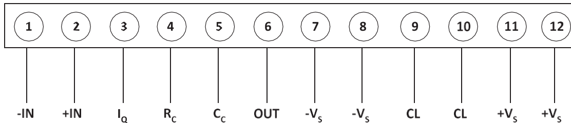
Figure 3: 外部接続図
