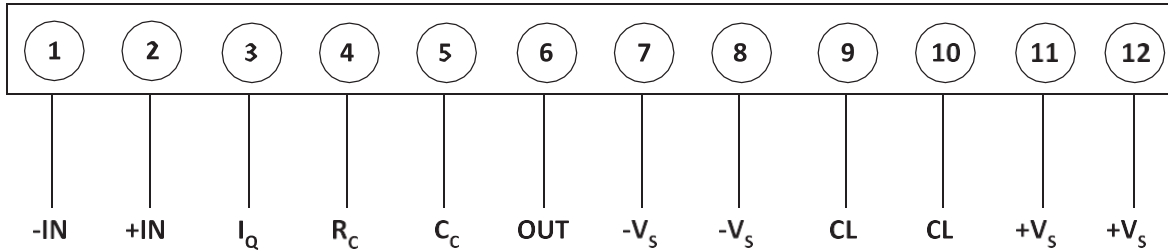
Figure 3: 外部接続図
