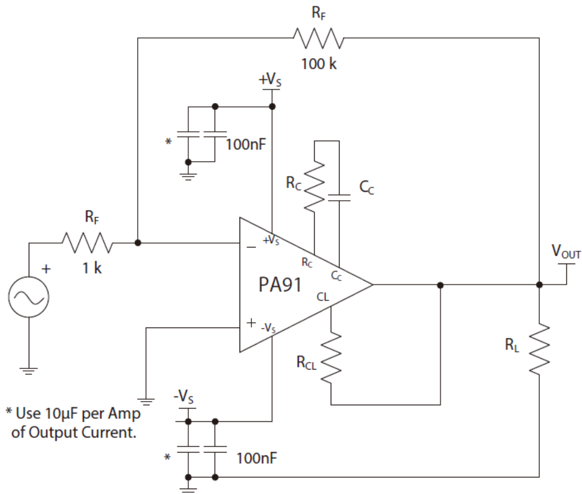
Figure 2: 代表的な接続図
