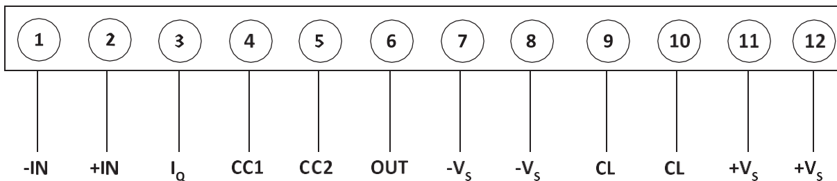
Figure 3: 外部接続図
